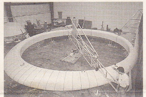
Die Mutterform des tragenden Rings in der endgültigen Fertigung.
